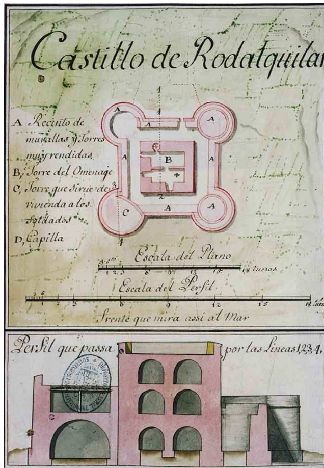
Planta y sección de la torre Fuerte o de los Alumbres de Rodalquilar. Sin fecha ni firma. A.G.M.M.: 3.035. B-8-2. 23/3
